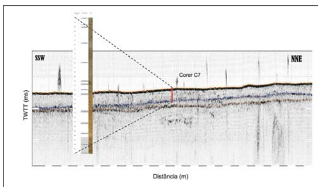
Fig. 2 – Perfil de sonar chirp ( sisch_07 ) onde se pode observar as duas sub-unidades acústicas superficiais. O testemunho C7 foi amostrado no centro geométrico da área de interesse e o seu comprimento total foi de 301 cm
