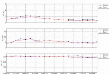
Fig. 3 – Comparação entre dados da bóia de Sines e o ponto respectivo do modelo SWAN local. Os dados do modelo correspondem a uma previsão a 24 horas
