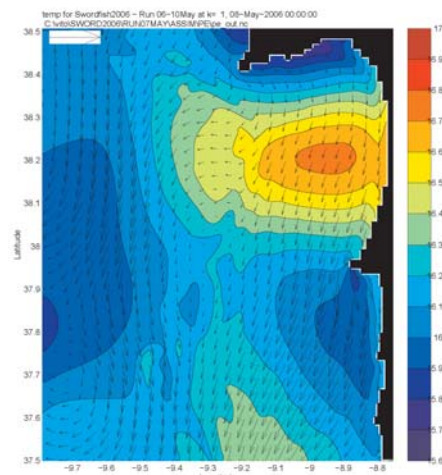
Fig. 5b – Previsão do modelo HOPS para a temperatura e velocidade à superfície em 8 de Maio
